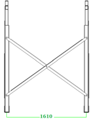
Resim 9: Sehpa Arkadan Görünüş
