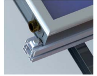
Resim 11: Alt Tutamak Sabitleme
